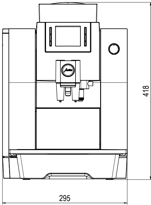
Framifrån
