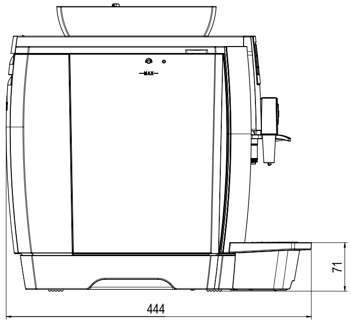
Från sidan
